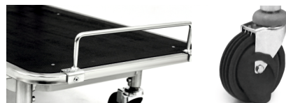
Zestaw elementów wymaganych do użycia wózka na chodnikach ruchomych (koła i ogranicznik frontowy):
